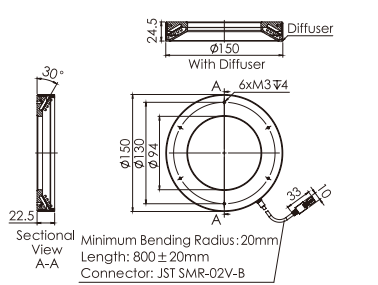
22.OPT-RI7045
