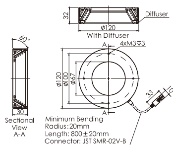
28.OPT-RI12060
