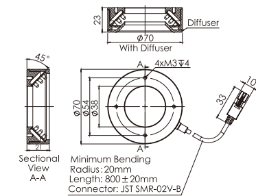
25.OPT-RI15045
