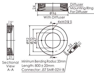
13.OPT-RI2825
