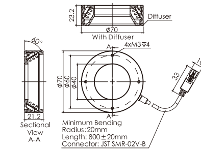
26.OPT-RI7060
