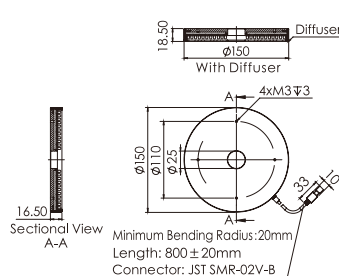
7.OPT-RI15000
