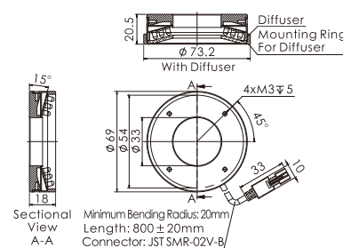
9.OPT-RI6915
