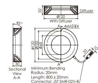
27.OPT-RI9060
