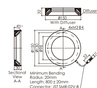
25.OPT-RI15045
