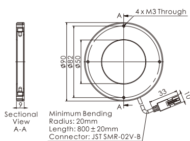
38.OPT-RI9090
