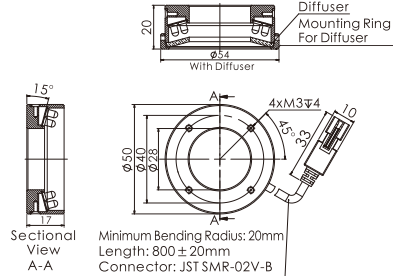
8.OPT-RI5015
