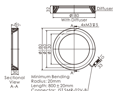
30.OPT-RI18060
