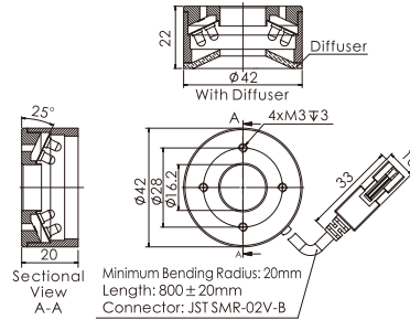
14.OPT-RI4225
