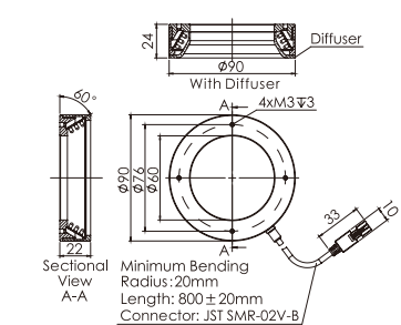
27.OPT-RI9060
