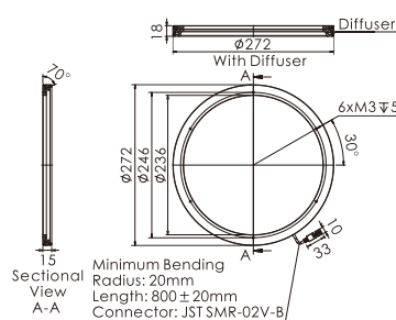
31.OPT-RI27270
