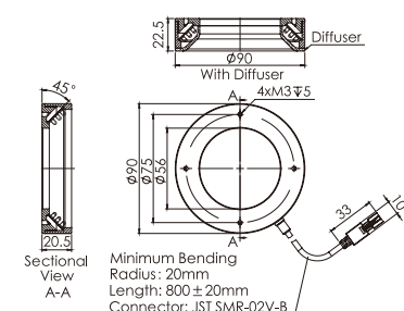
26.OPT-RI7060
