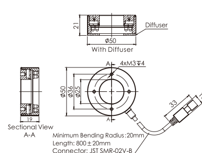
3.OPT-RI5000
