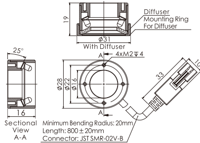
13.OPT-RI2825
