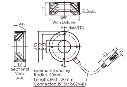
24.OPT-RI12045
