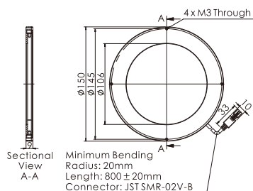
40.OPT-RI15090
