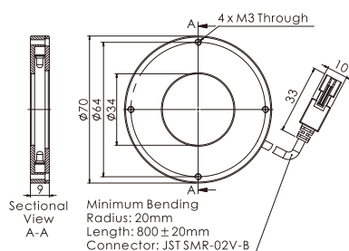
37.OPT-RI7090
