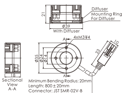
2.OPT-RI3500
