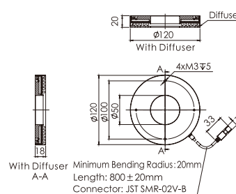
6.OPT-RI12000
