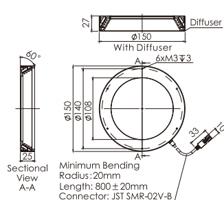
29.OPT-RI15060
