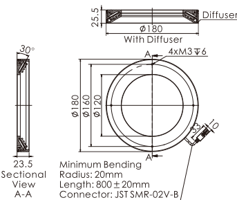
23.OPT-RI9045
