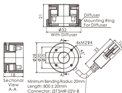
1.OPT-RI2800
