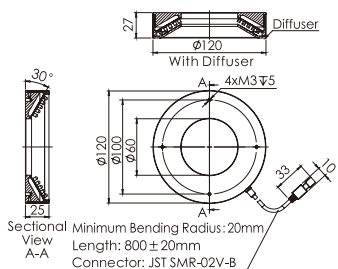
21.OPT-RI5045
