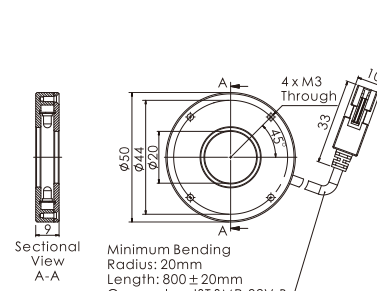
36.OPT-RI5090
