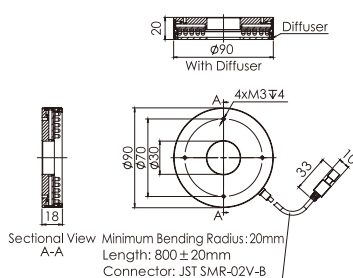
5.OPT-RI9000
