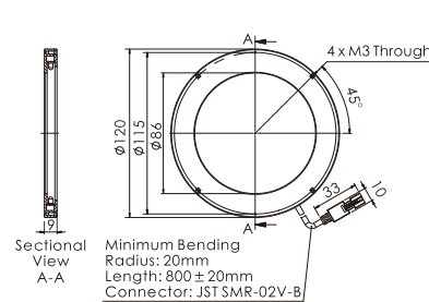
39.OPT-RI12090
