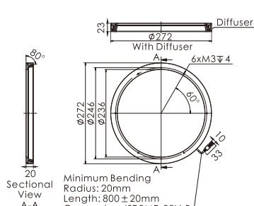
35.OPT-RI27280
