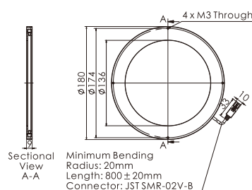
41.OPT-RI18090
