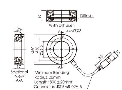
18.OPT-RI12030
