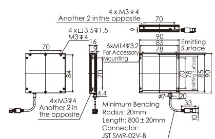
6.OPT-FL9090
