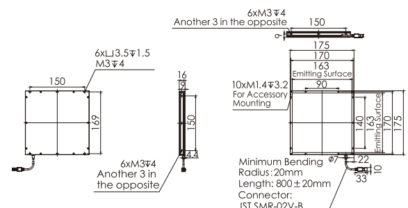
10.OPT-FL175175
