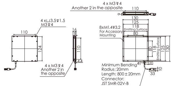
8.OPT-FL130130
