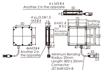
5.OPT-FL7070
