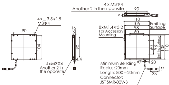
7.OPT-FL110110
