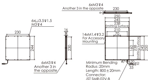
13.OPT-FL250250
