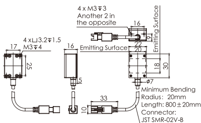
1.OPT-FL3022
