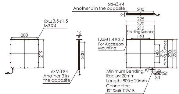
12.OPT-FL225225
