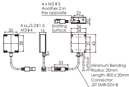
2.OPT-FL4336
