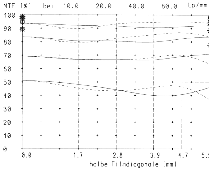
Modulationstransferfunktion bei M = 0.05x Blende 1.8
