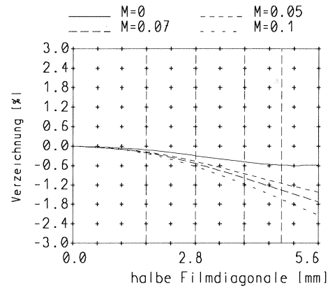
Verzeichnung bei M = 0 bis M = 0.1
